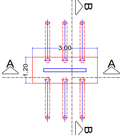
Planta Sapata S5 Esc.: 1/100
