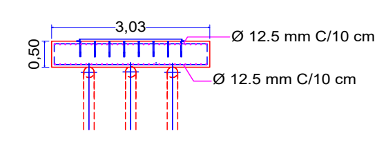
Corte A-A S5 Esc.: 1/100
