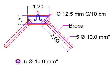
Corte B-B S5 Esc.: 1/100
