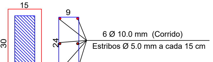
VR Vigas Respaldo (15 x 30 cm) Escala.: 1:10
