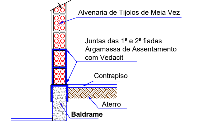
Det. Impermeabilização nos Alicerces S/Escala
