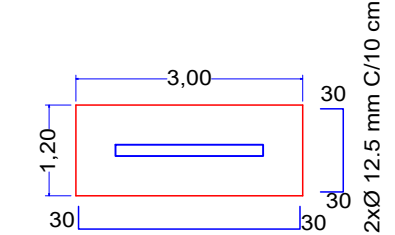
Ferragem S5 Esc.: 1/100
