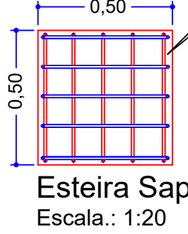
Sapata S2 Escala.: 1:20
