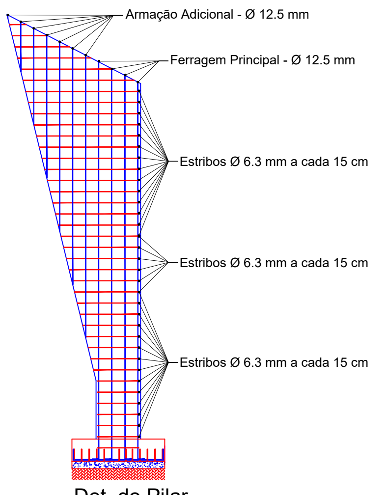
Det. do Pilar Escala.: 1:50
