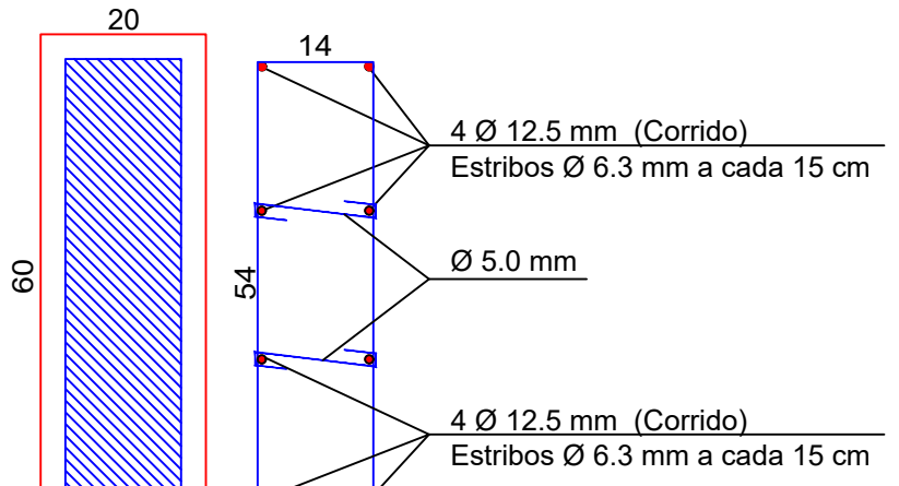
P2 Pilares (20 x 60 cm) Escala.: 1:10
