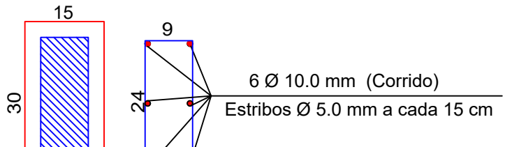
VB Vigas Baldrame (15 x 30 cm) Escala.: 1:10
