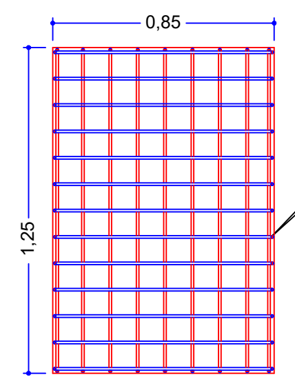
Esteira Sapata S4 Escala.: 1:20
