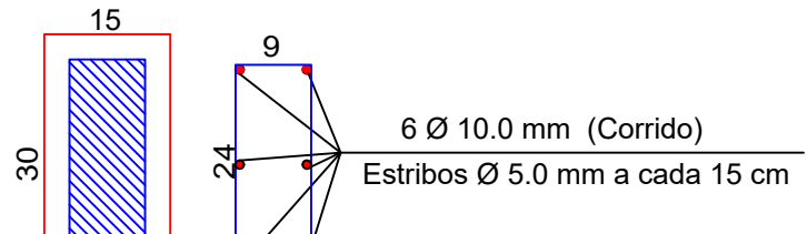
P1 Pilares (15 x 30 cm) Escala.: 1:10
